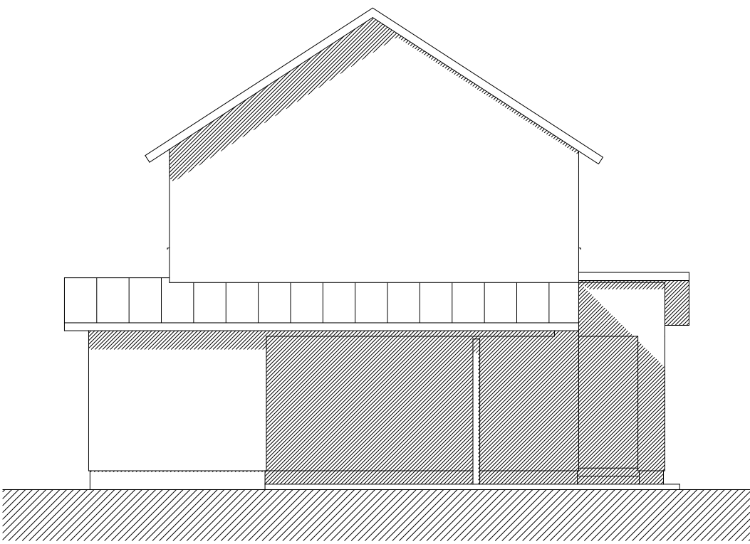
Julkisivu Itään
