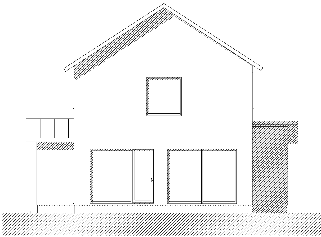
Julkisivu Länteen
