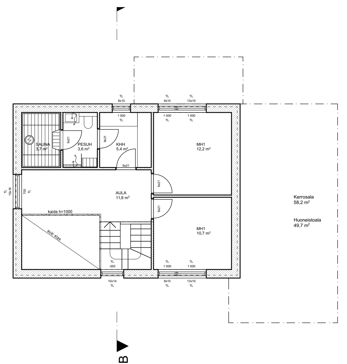
2. Kerros (5)
