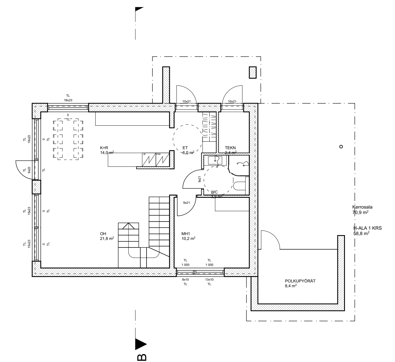
ARK 02 - POHJA
